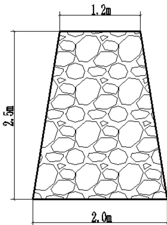
图 3.5-1 1#排土场下游拦挡墙
