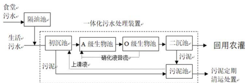
图 14.2-1 生活污水处理站工艺流程图
